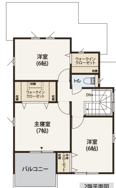
2階平面図
