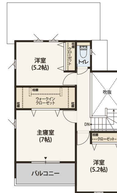
2階平面図
