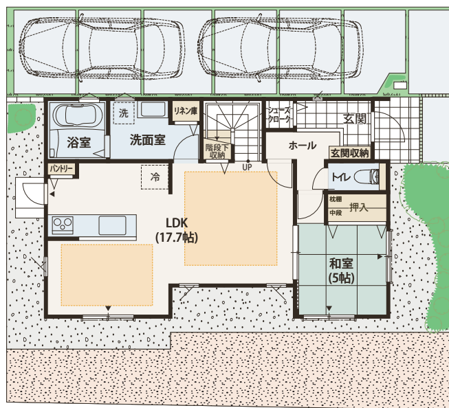
1階平面図
