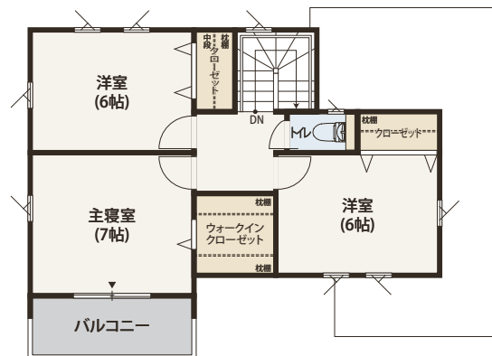
2階平面図
