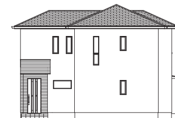
北側立面図
