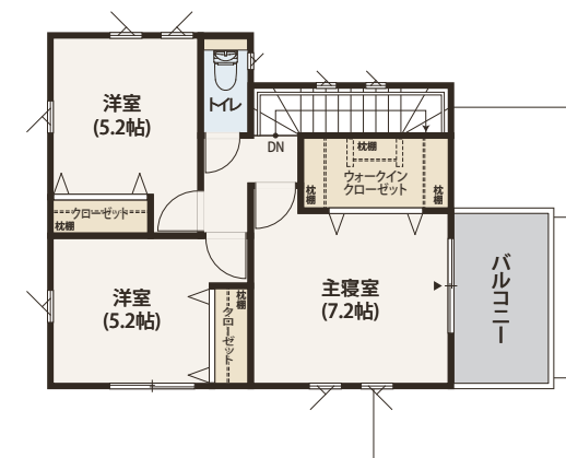
2階平面図
