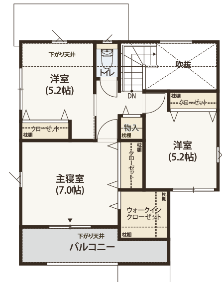
2階平面図
