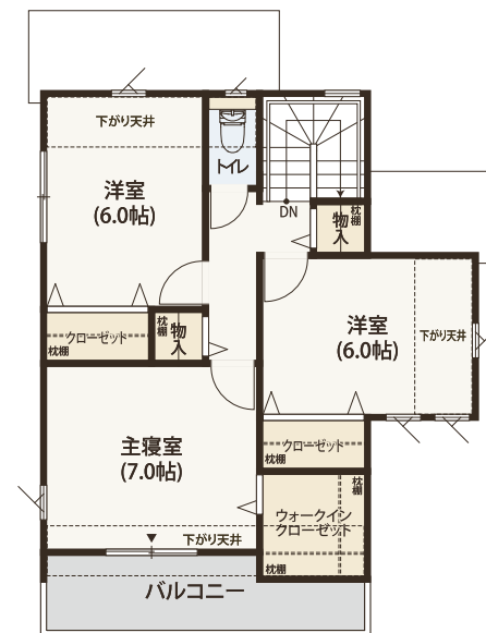
2階平面図
