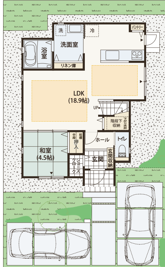
1階平面図
