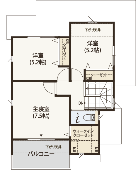
2階平面図
