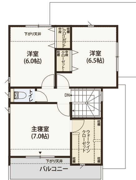
2階平面図
