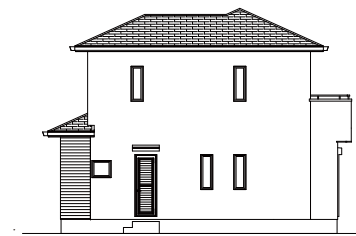
西側立面図
