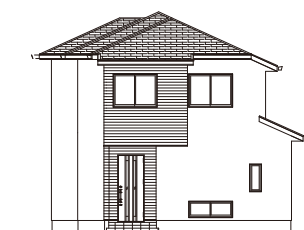
東側立面図
