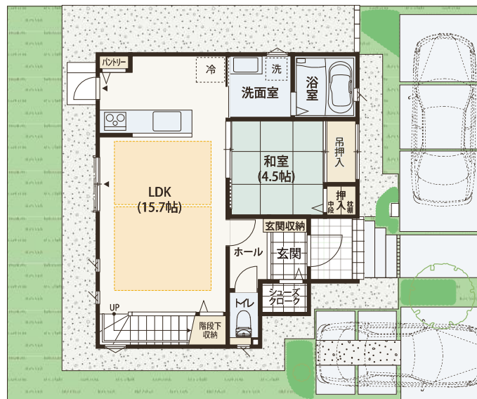
1階平面図
