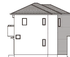
南側立面図
