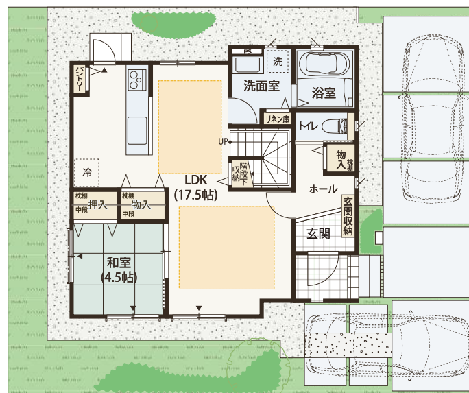
1階平面図
