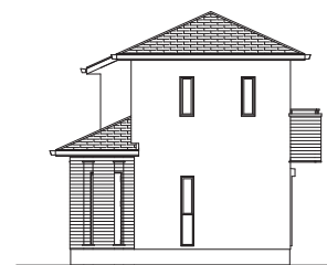
西側立面図
