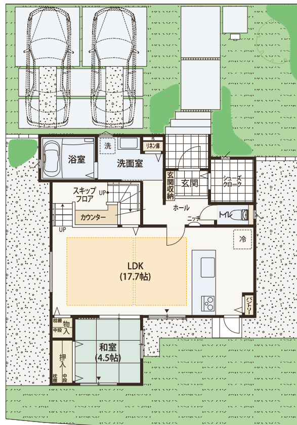
1階平面図
